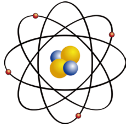
Borsches Atommodell. Die Elektronen umkreisen den Atomkern, der aus Protonen und Neutronen besteht. Es gibt immer die gleiche Zahl an negativ geladenen Elektronen und positiv geladenen Protonen. Grafik: Dario Sabljak
